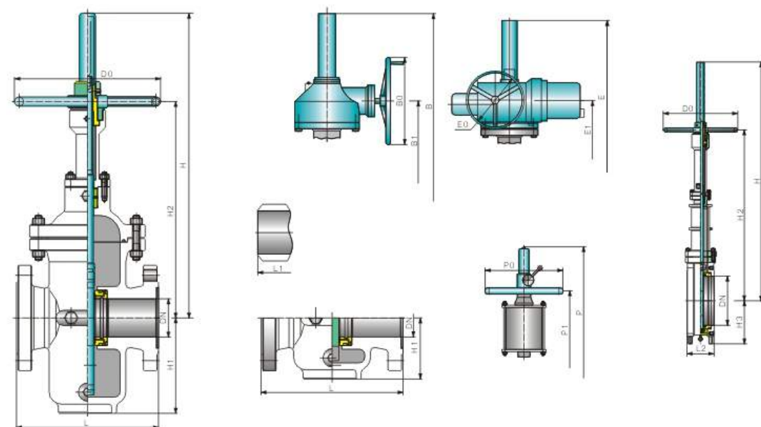
● 主要外形尺寸及重量 Main size of outside & weight 型号 Model: (K)Z5(6、9)4(6)3(4)W(P)(F、Y、D)PN6.4MPa (Class400)
