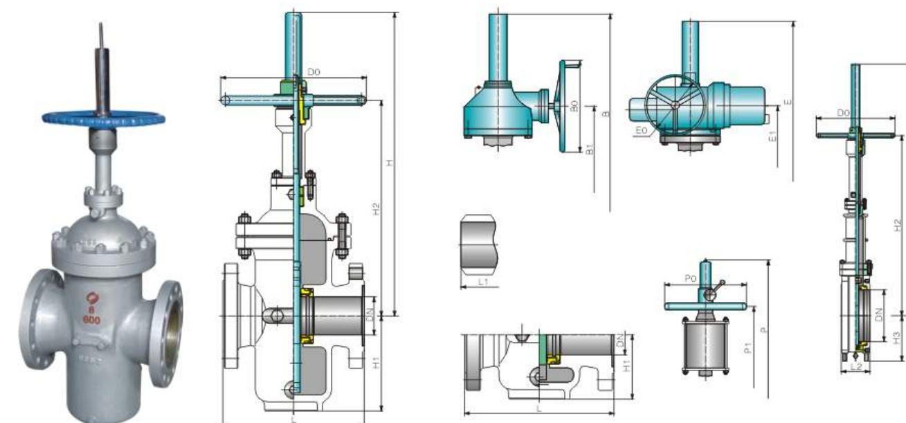
●主要外形尺寸及重量 Main size of outside & weight 型号 Model: (K)Z5(6、9)4(6)3(4)W(P)(F、Y、D)PN10.0MPa (Class600)
