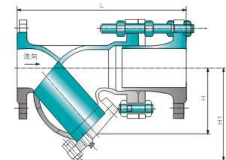
YSTF型拉杆伸缩过滤器
