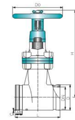
SJKSZ(带信号软密封闸阀) SJKIZ(带开度指示软密封闸阀)
