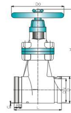
SJKHZ(非升杆式软密封闸阀)
