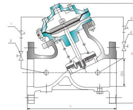
1、过滤器 2、小球阀 3、过滤器 4、小球阀
