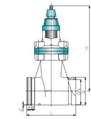
SJKCZ(附传动帽非升杆式软密封闸阀)
