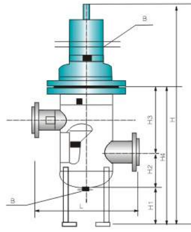
SBL封头式
