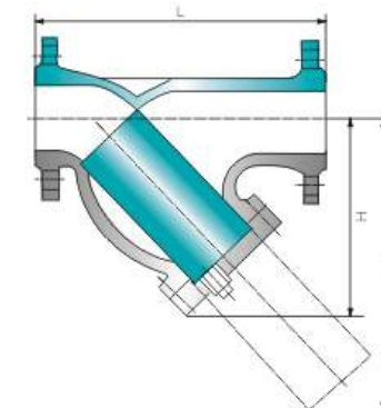
SY4P型过滤器
