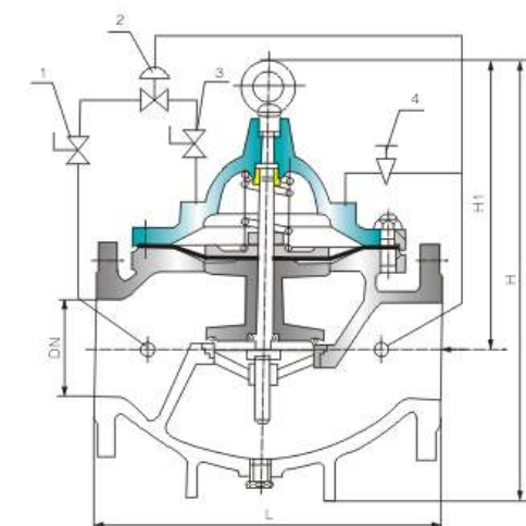
1、小球阀 2、导阀 3、小球阀 4、针型阀
