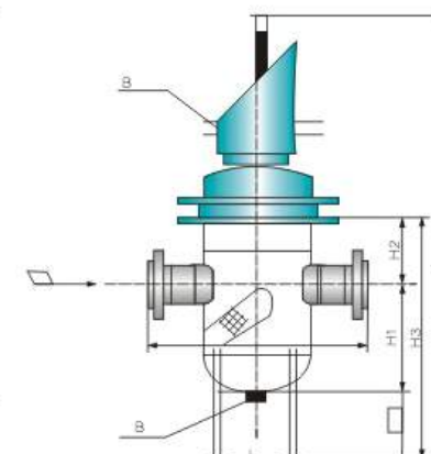
SBL封头式
