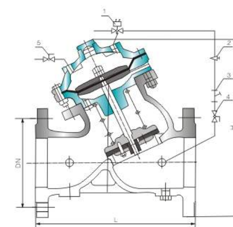
1、电磁导阀 2、针型阀 3、过滤器 4、小球阀 5、小球阀
