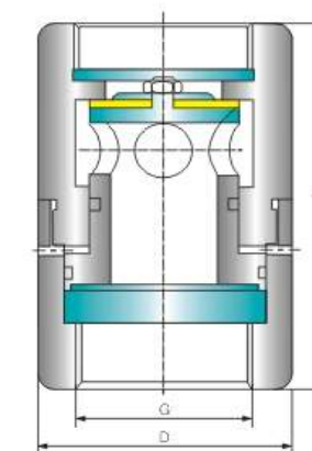
YB13X-10/16 T(B型)
