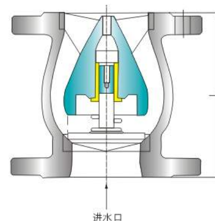
进水口
