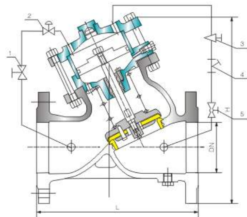
1、小球浮阀 2、导阀 3、针型阀 4、过滤器 5、小球阀
