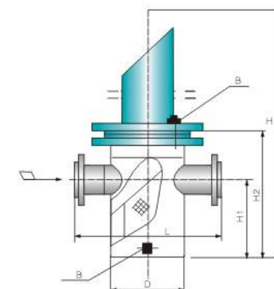
SBL平底式
