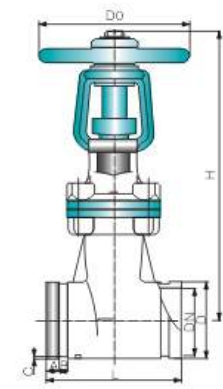
SJKRZ(升杆式软密封闸阀)
