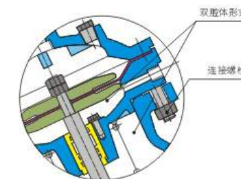
双阀腔示意图
