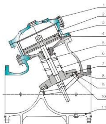
BYH103X活塞式遥控浮球阀 BYH104X活塞式可调减压稳压阀 BYAX107X活塞式安全泄压/持压阀 BYH108X活塞式电动遥控阀
