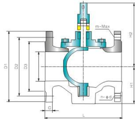
DN20~200结构
