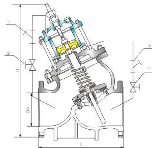
1、过滤器 2、小球阀 3、过滤器 4、小球阀
