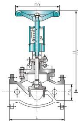
TJ40型
