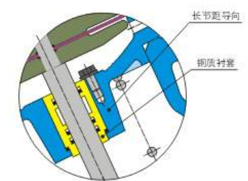
阀杆导向示意图
