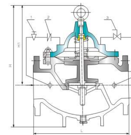
1、针形阀 2、止回阀 3、小球阀
