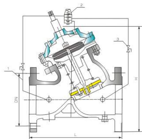
1、小球阀 2、导阀 3、小球阀
