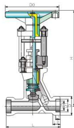
WJ61型
